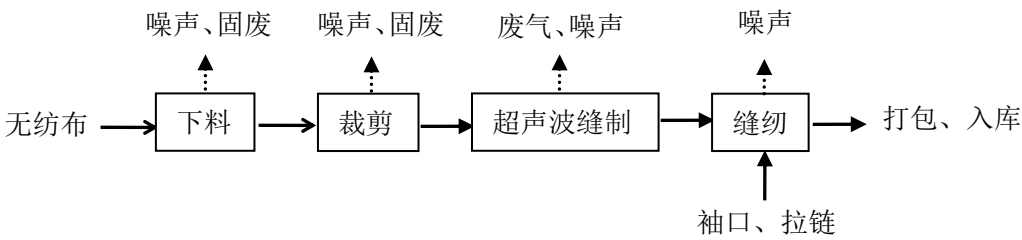
图4 防护服生产工艺流程和产污环节示意图
