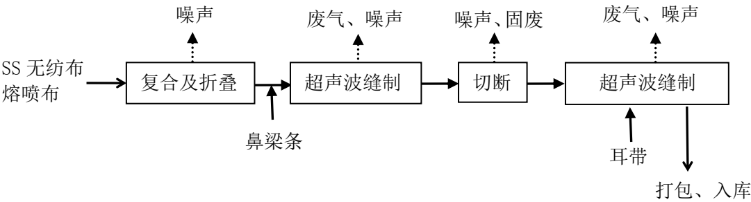
图3 一次性口罩生产工艺流程和产污环节示意图
