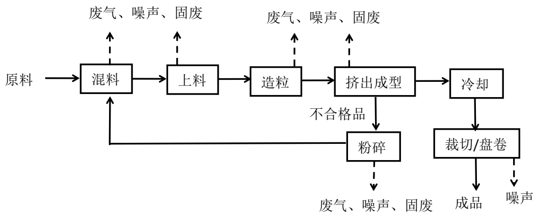
图 3 生产工艺流程及排污节点图
