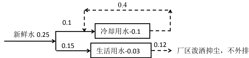
图 1 项目水平衡图 单位 m 3 /d
