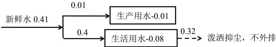
图 1 项目水平衡图 单位 m³/d
