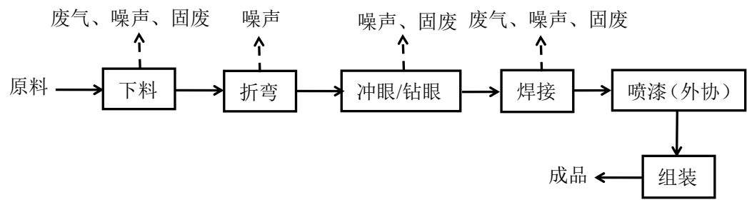
图 4 生产工艺流程及排污节点图
