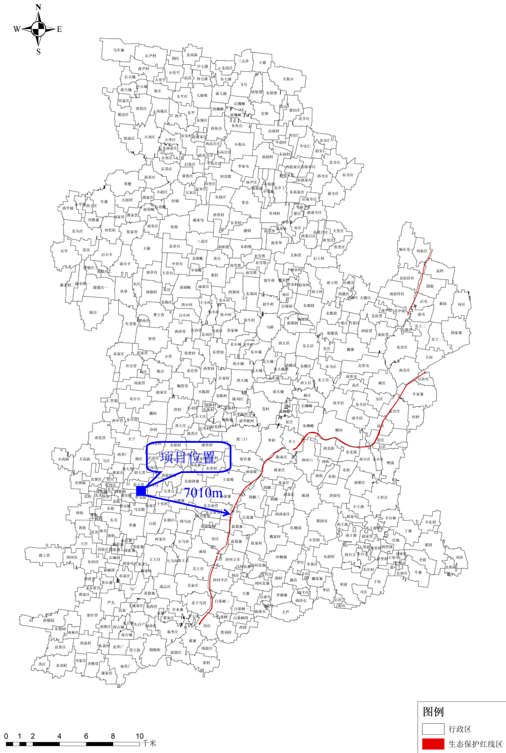
图2 威县生态保护红线区分布图
